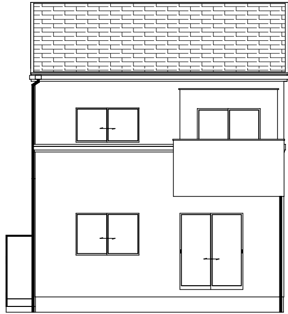
南側 立面図
