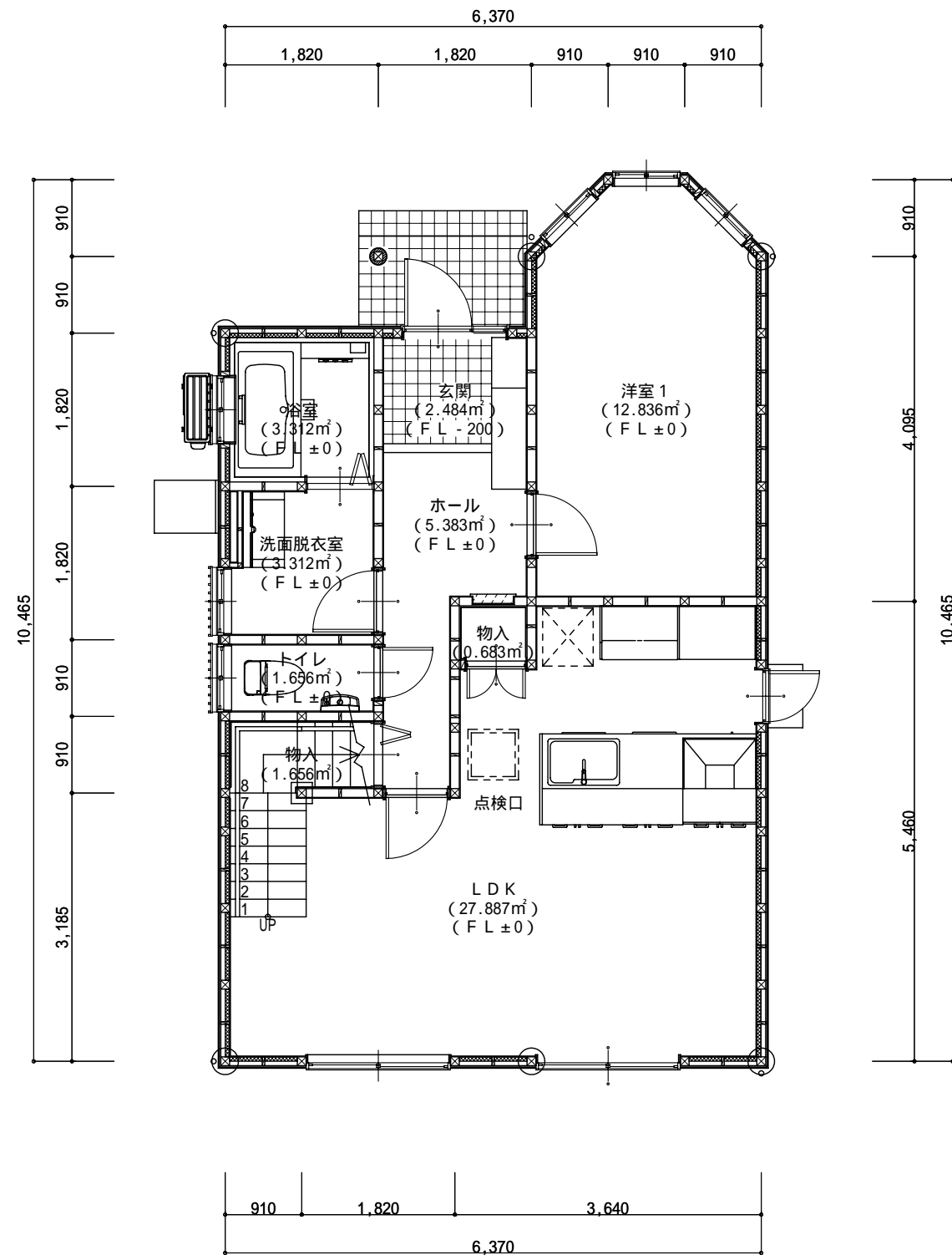
1階 平面図
