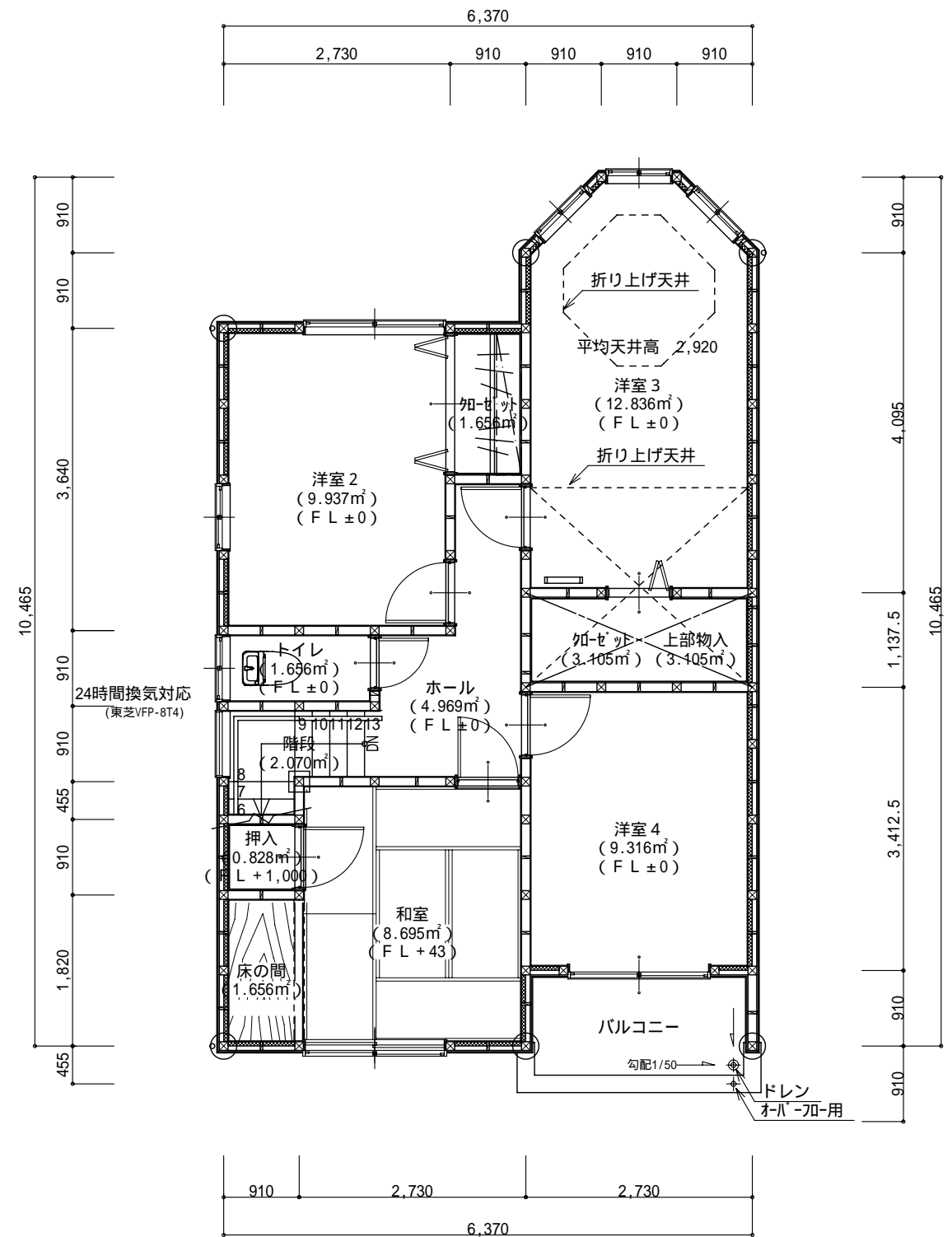
2階 平面詳細図 S:1/75
