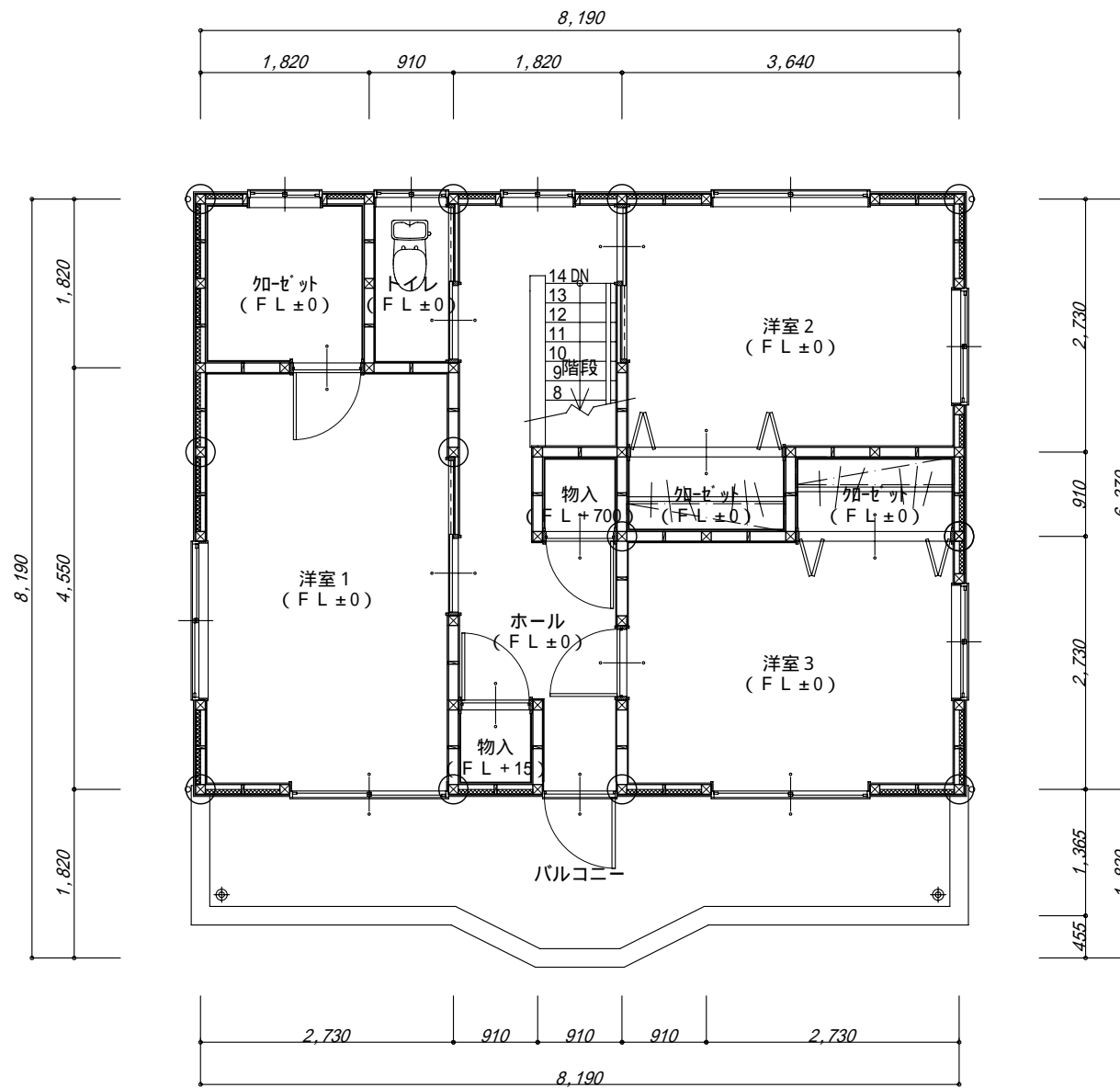
2階 平面図
