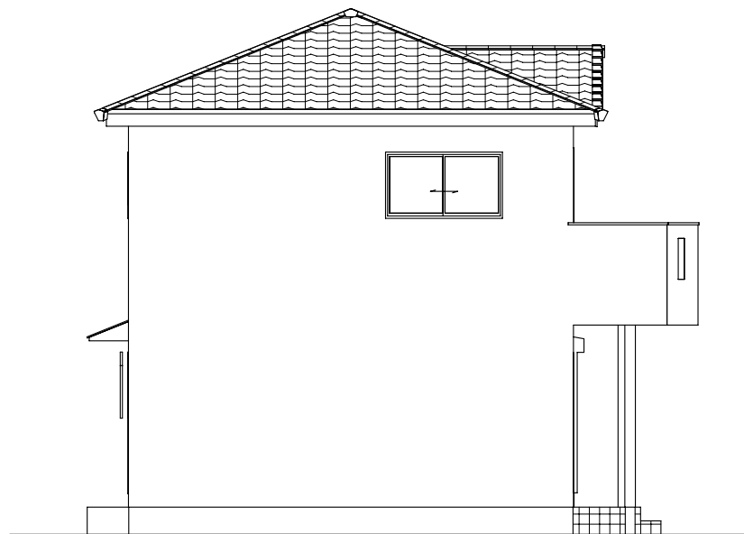
西側 立面图
