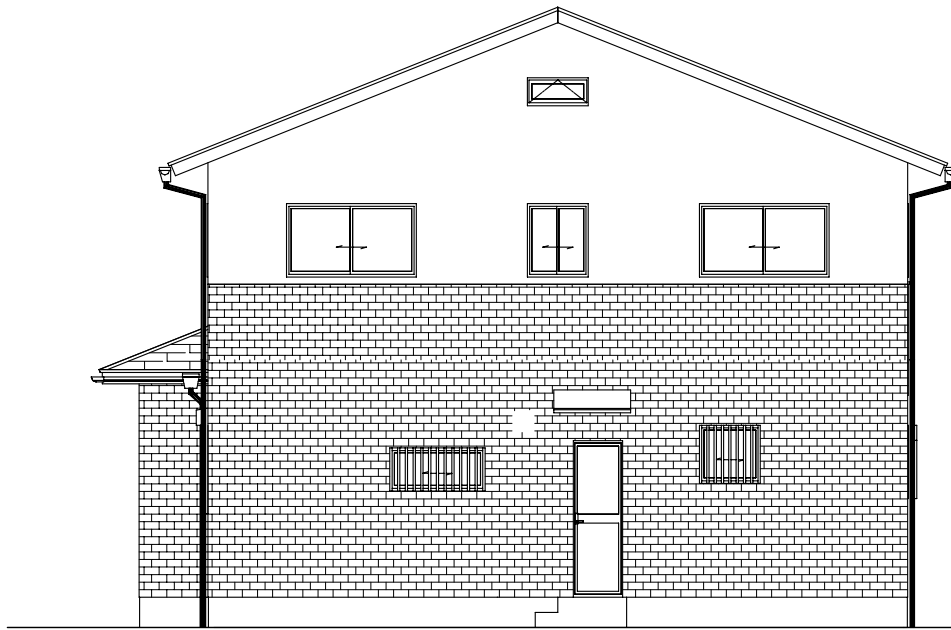
北側 立面図
