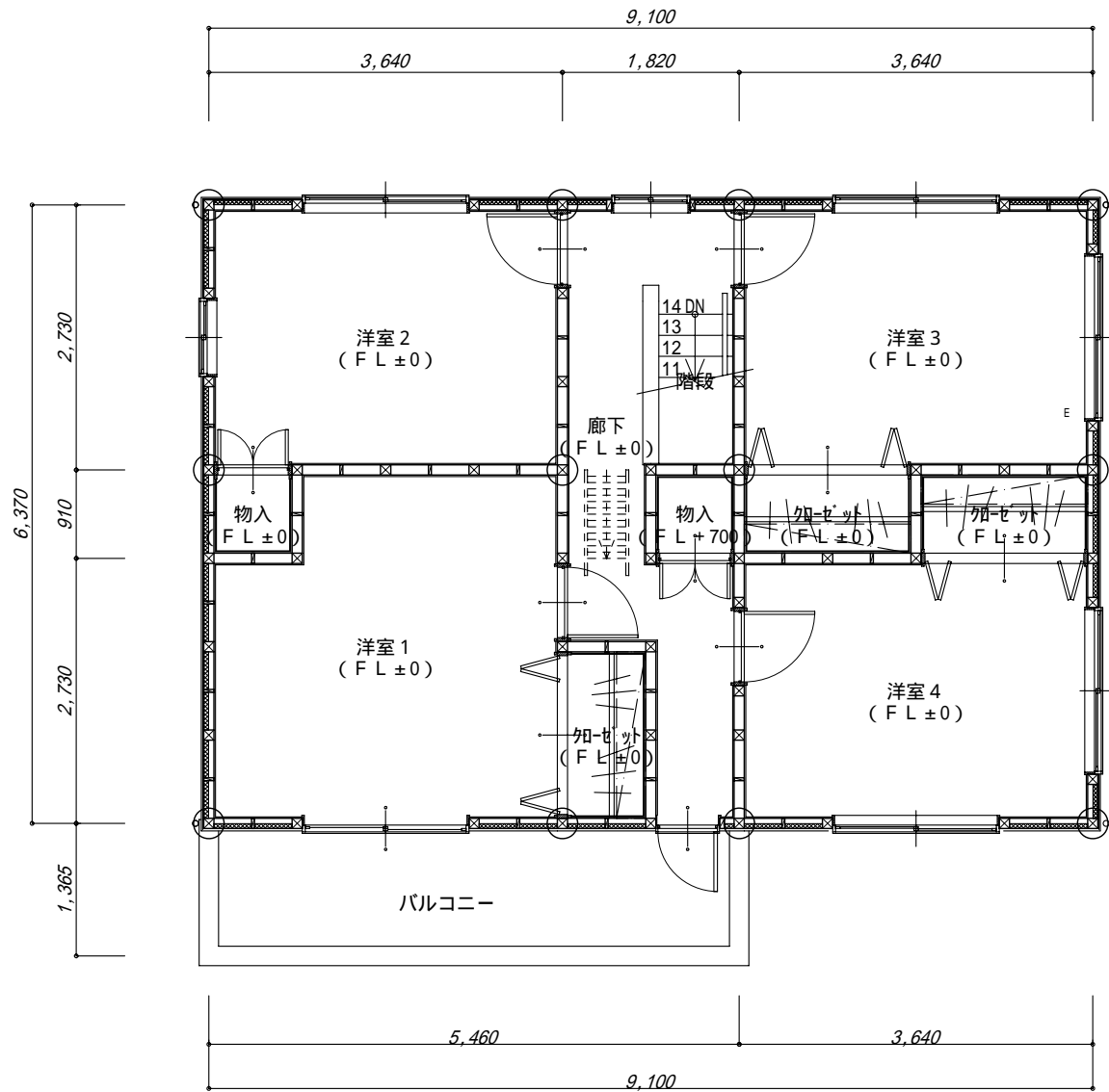
2階 平面図
