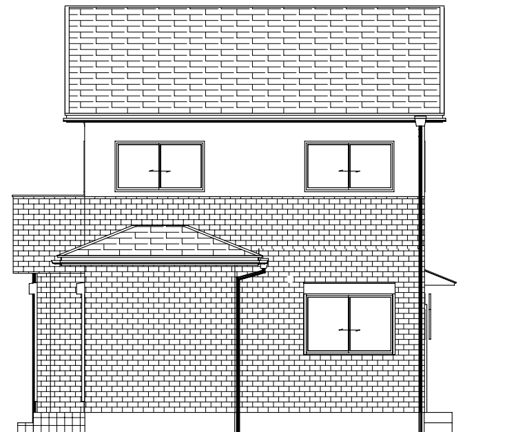
東側 立面図
