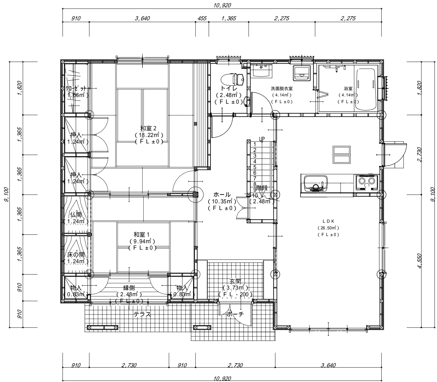
1階 平面図
