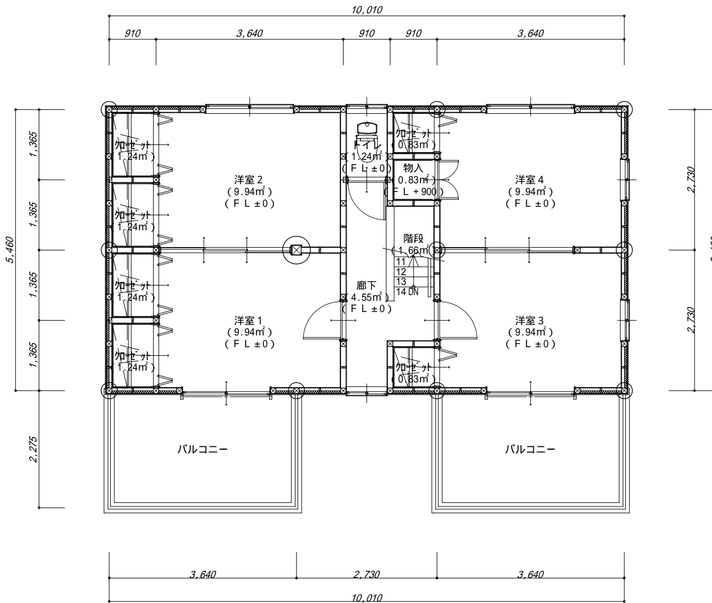
2階 平面図
