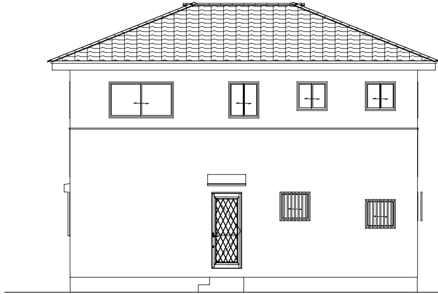
北側 立面図
