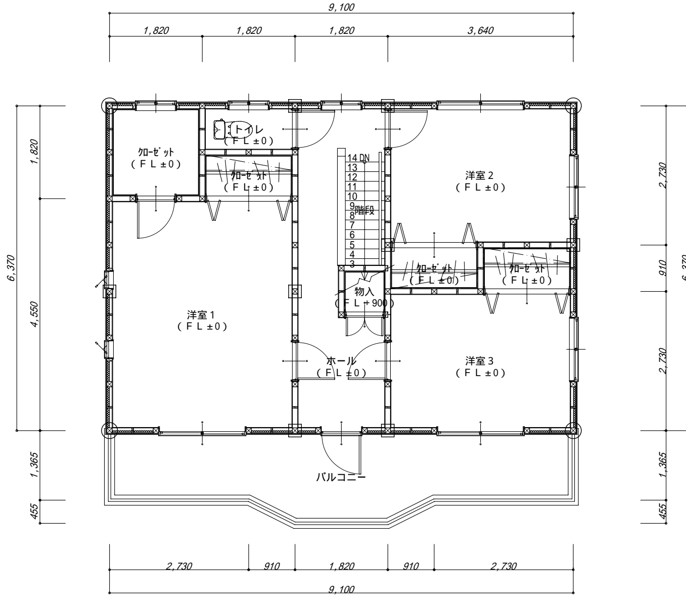
2階 平面図
