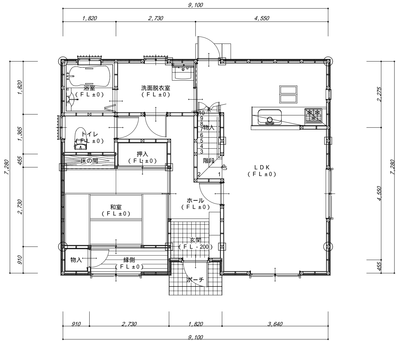
1階 平面図
